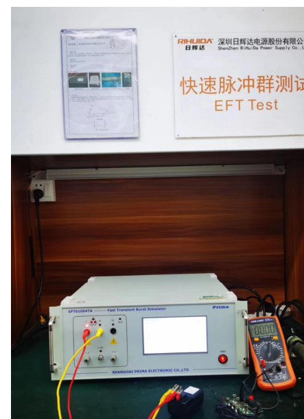
快速脉冲群
